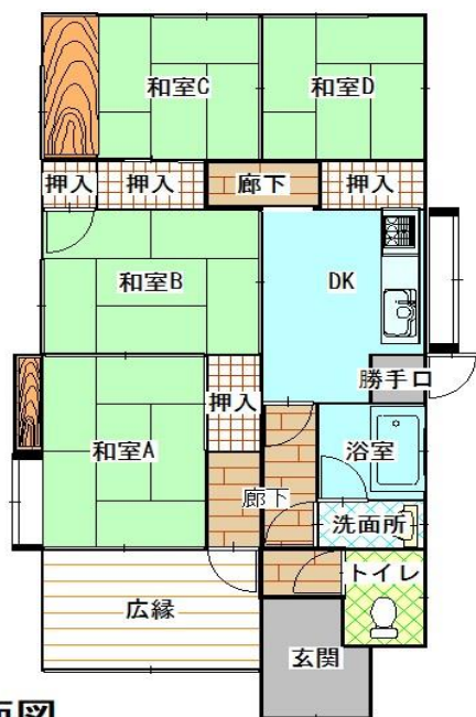
平面図
