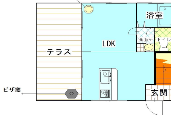
1階平面図
