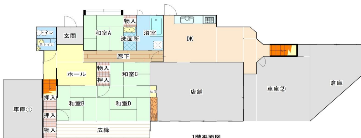
1階平面図
