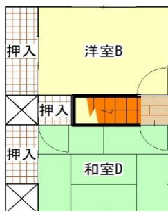
2階平面図
